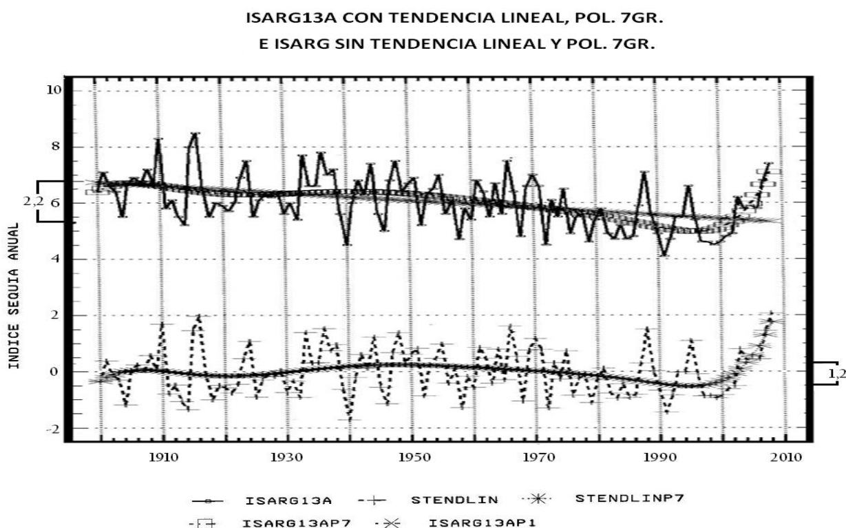
Figura 1: Índice de sequía anual en Argentina con y sin tendencia 1901-2010
