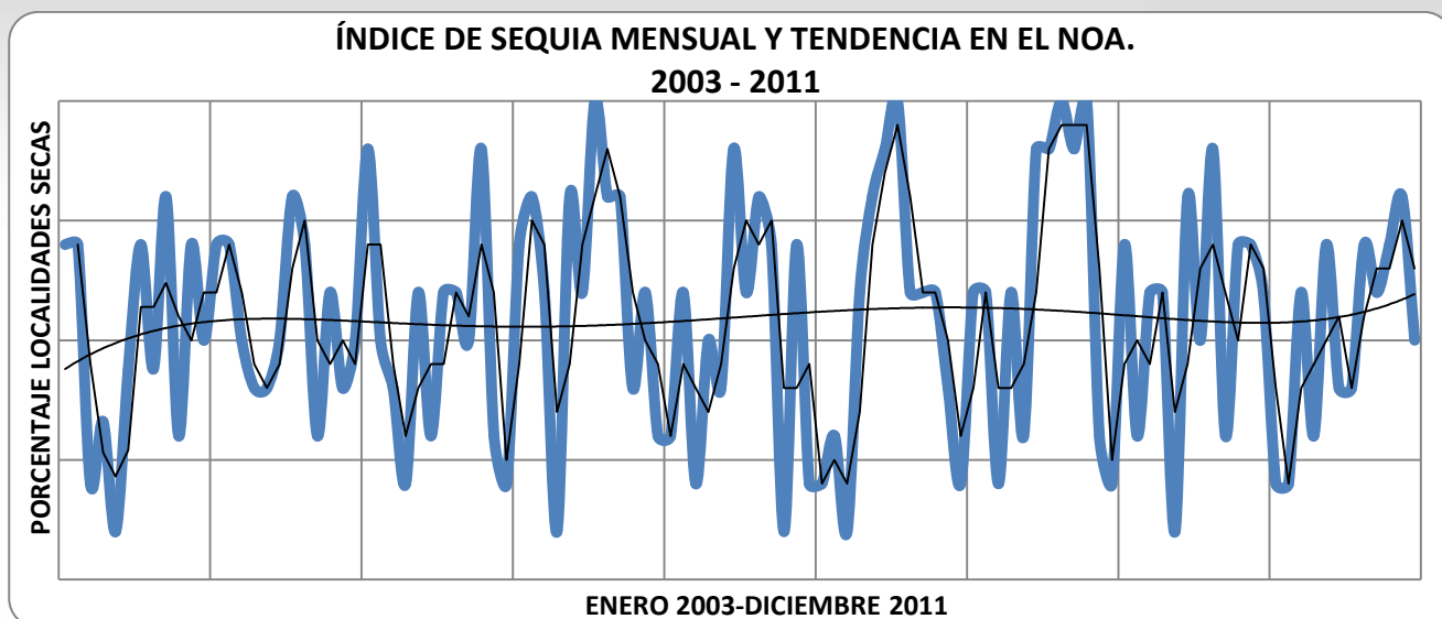
Figura 3: Índice de sequía mensual y tendencia en el NOA 2003-2011.
